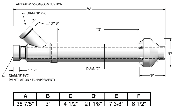
Figure 3-9 Schéma des dimensions de ventilation concentrique - Modèles 126-065 -- 201-100 / 100140480
