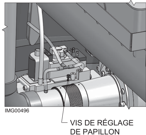
Figure 12-3 Réglage du robinet de gaz: Modèle 401-125
