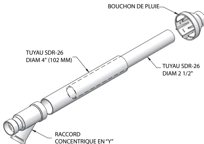
Figure 3-8 Contenu du kit_100140484- 286-125 -- 501-125
