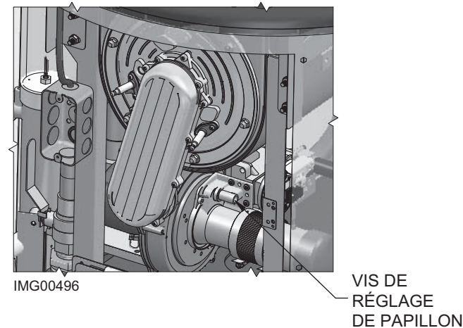
Figure 12-2 Réglage du robinet de gaz: Modèles 126-065 -- 286-125
