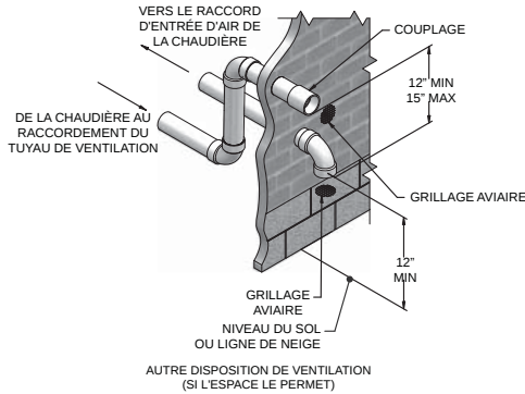
Figure 3-1D Alternar la disposition de ventilation SS Terminaison d'air murale classique en acier inoxydable et ventilation avec raccords fournis sur place, utilisant une entrée capot
