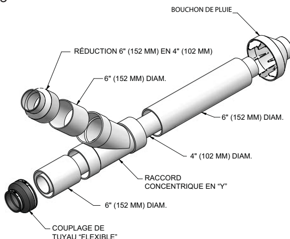
Figure 3-8 Contenu du kit_100140484- 286-125 -- 501-125
