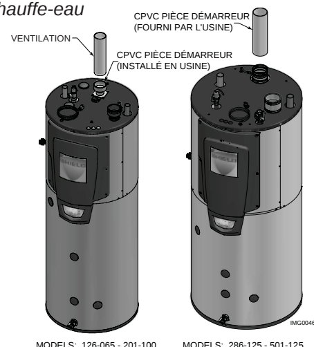
Figure 2-7 Près de la ventilation en PVC/CPVC du chauffe-eau
