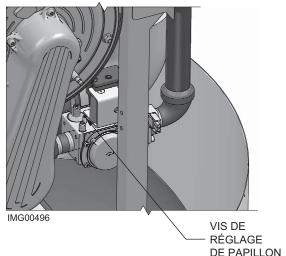
Figure 12-4 Réglage du robinet de gaz: Modèle 501-125
