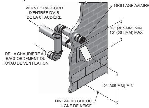
Figure 3-1D Alternar la disposition de ventilation SS Terminaison d'air murale classique en acier inoxydable et ventilation avec raccords fournis sur place, utilisant une entrée capot
