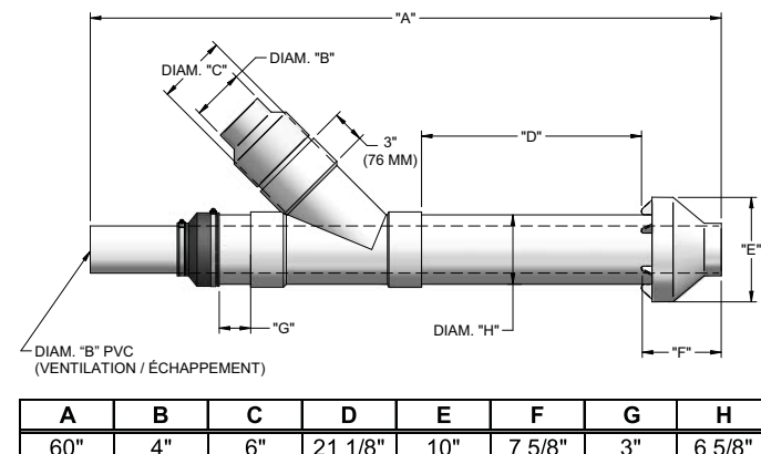
Figure 3-10 Schéma des dimensions de ventilation concentrique - Modèles 286-125 -- 501-125 / 100140484
