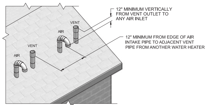
Figure 4-3 Terminaisons verticales alternatives avec chauffe-eaus multiples
